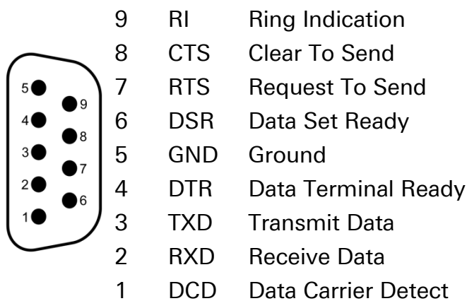
Abbildung 5: Belegung RS232-Schnittstelle
