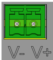
Abbildung 4: SCR – Anschluss Spannungsversorgung
