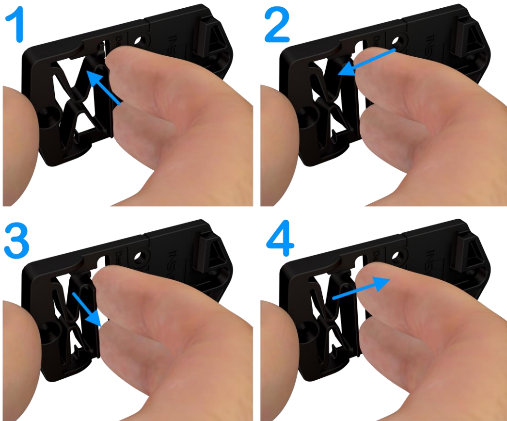
Abbildung 13: Hutschienenmontage– Vorspannen des Hutschienen-Adapters
