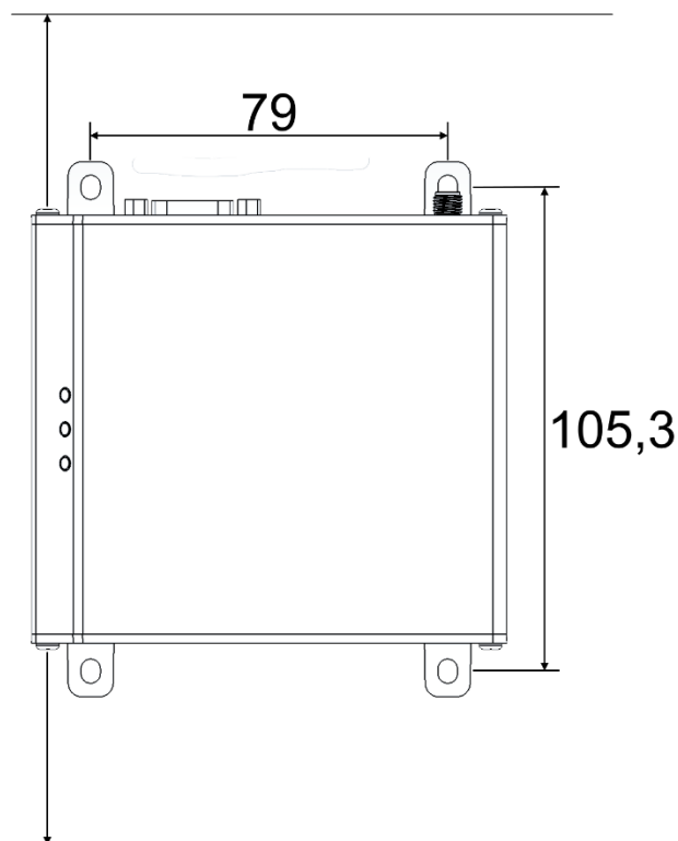
Abbildung 14: SCR – Abmessungen – Schraubmontage
