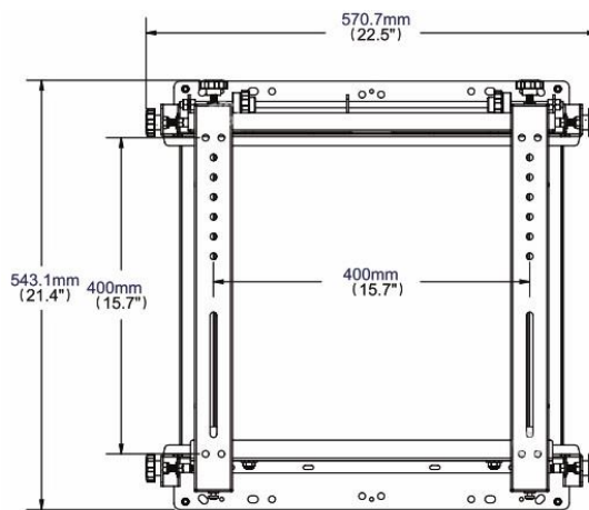
TiefenEinstellung an allen vier Ecken / Höheneinstellung an zwei Punkten
